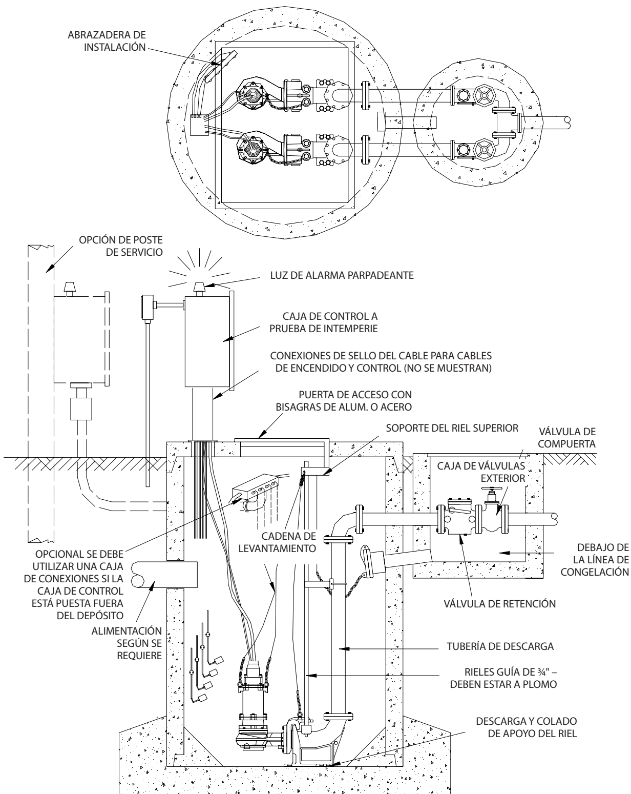
Figura 2 INSTALACIÓN TÍPICA PARA UN SISTEMA DÚPLEX CON DEPÓSITO DE HORMIGÓN Y CAJA DE VÁLVULAS EXTERIOR
